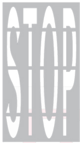
DIMA STOP EXTRAURBANO SIMBOLO ALTEZZA CM.400 DIMENSIONE DIMA COMPLETA CM. H. 420x232 SCRITTA FATTA CON 4 DIME
